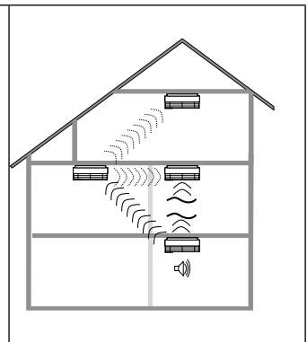
Abb. 03 Bei gestörter Funkstrecke übernimmt automatisch ein anderer Funk-Rauchwarnmelder die Repeaterfunktion, um eine flächendeckende Alarmierung sicherzustellen.
